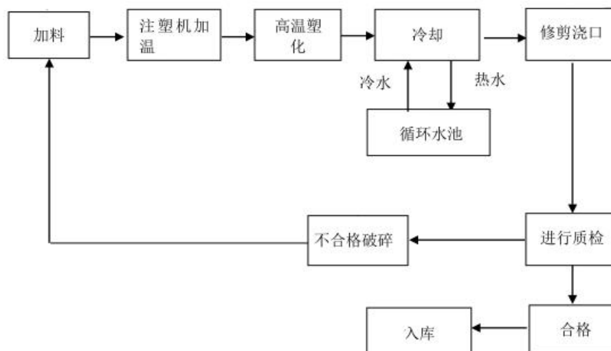
图 3-3 管件生产工艺流程图
