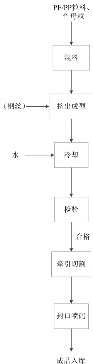
图 3-2 管材生产工艺流程图
